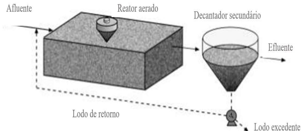
Figura 2. Esquema do tratamento por lodo ativado convencional Fonte: Sperling, 2014.
