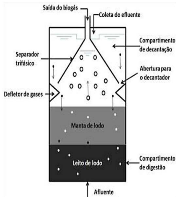
Figura 3. Esquema representativo do funcionamento de um reator UASB
